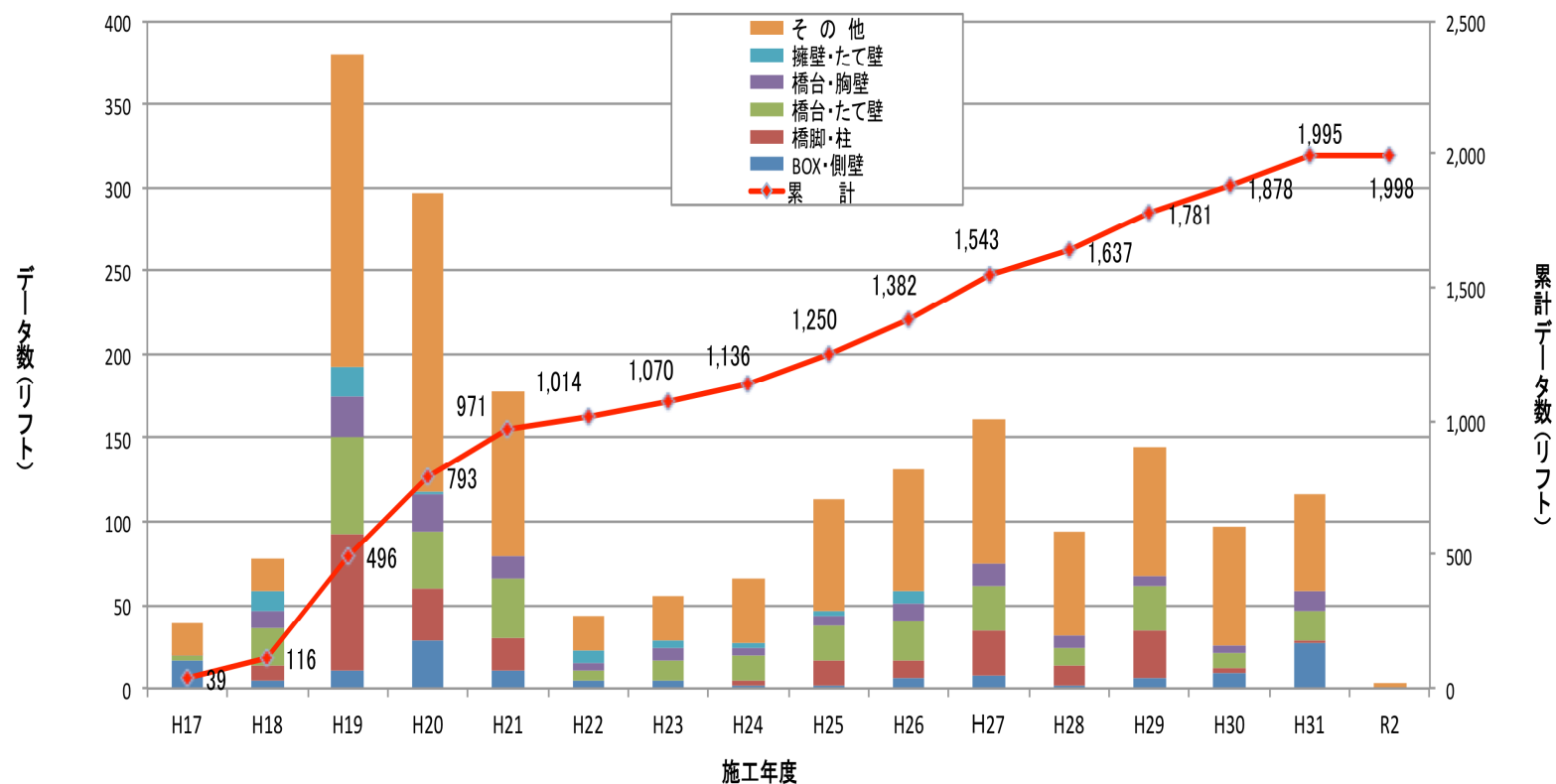
【コンクリート施工記録データ集計表(令和3年3月現在)】
